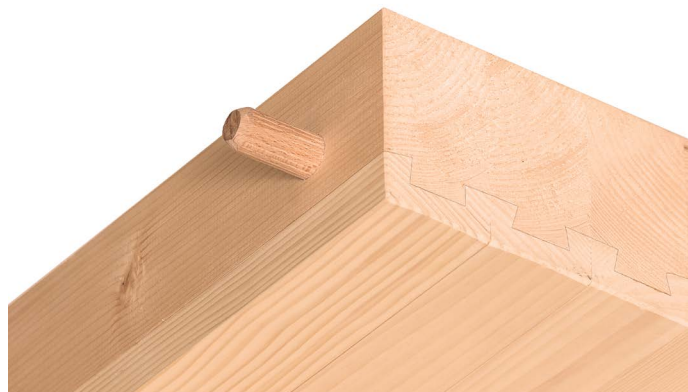
Schwalbenschwanzverbindung
